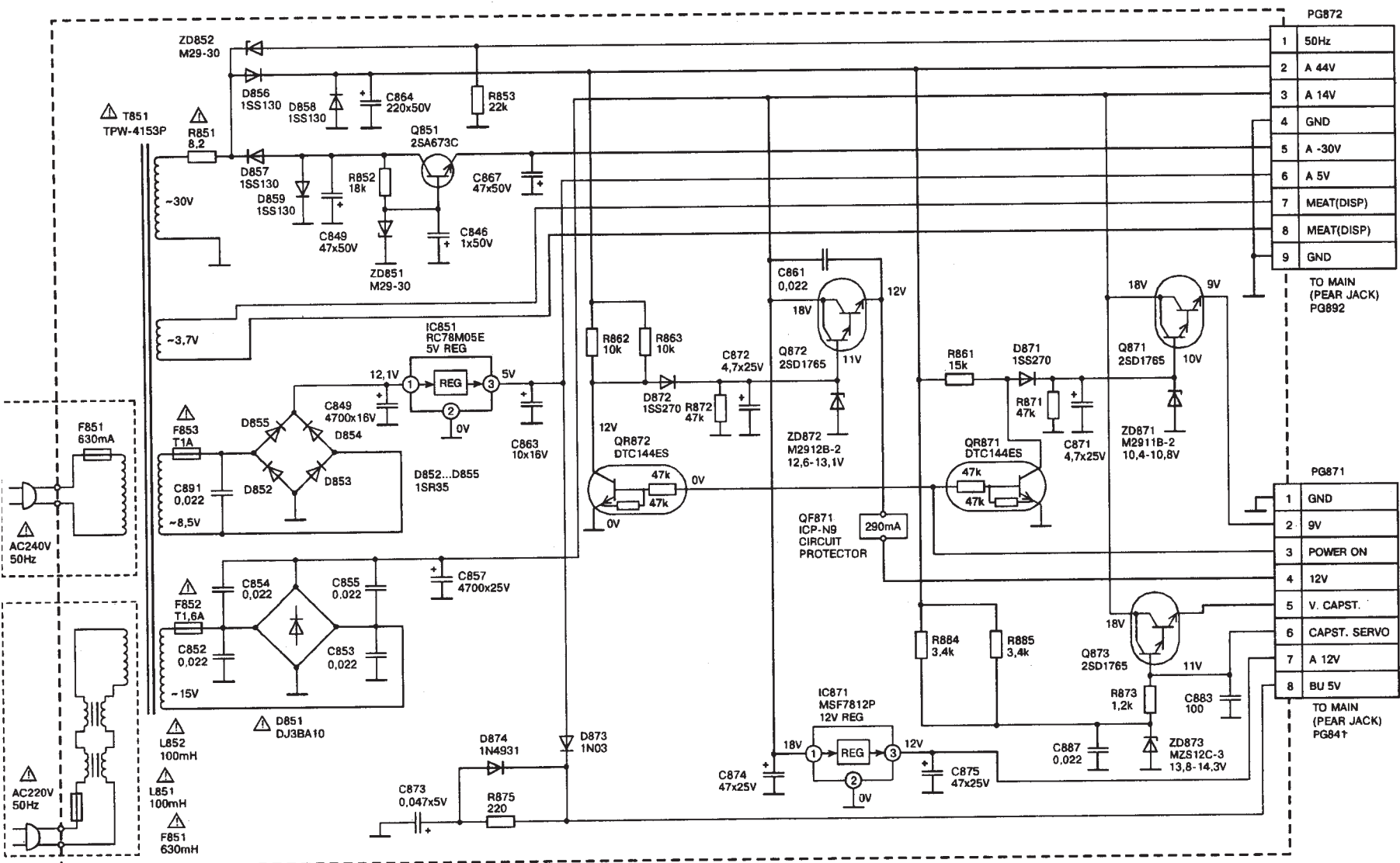
Принципиальная схема источника питания видеомэгафонов VT-M747GK/AU/UK
